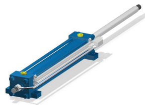
Zylinder mit Wegmesssystem aussen
