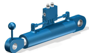
Zylinder mit Senkbremshalteventil
