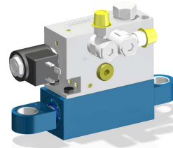
Steuerblockzylinder mit 4/2 Wegeventil und Senkbremshalteventil
